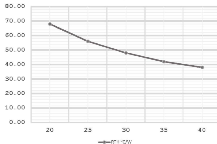
length (mm) vs R TH (°C/Watt)
