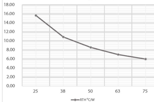
length (mm) vs R TH (°C/Watt)
