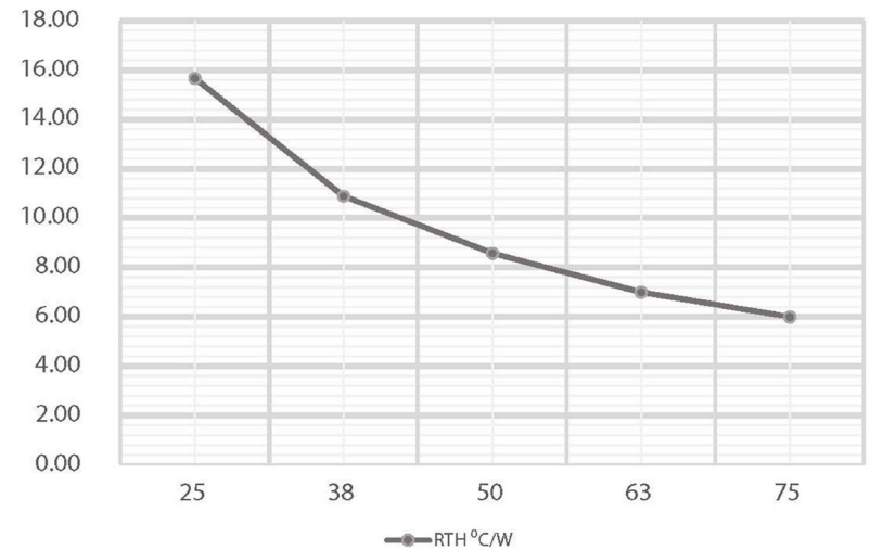
length (mm) vs R_{TH} (°C/Watt)
